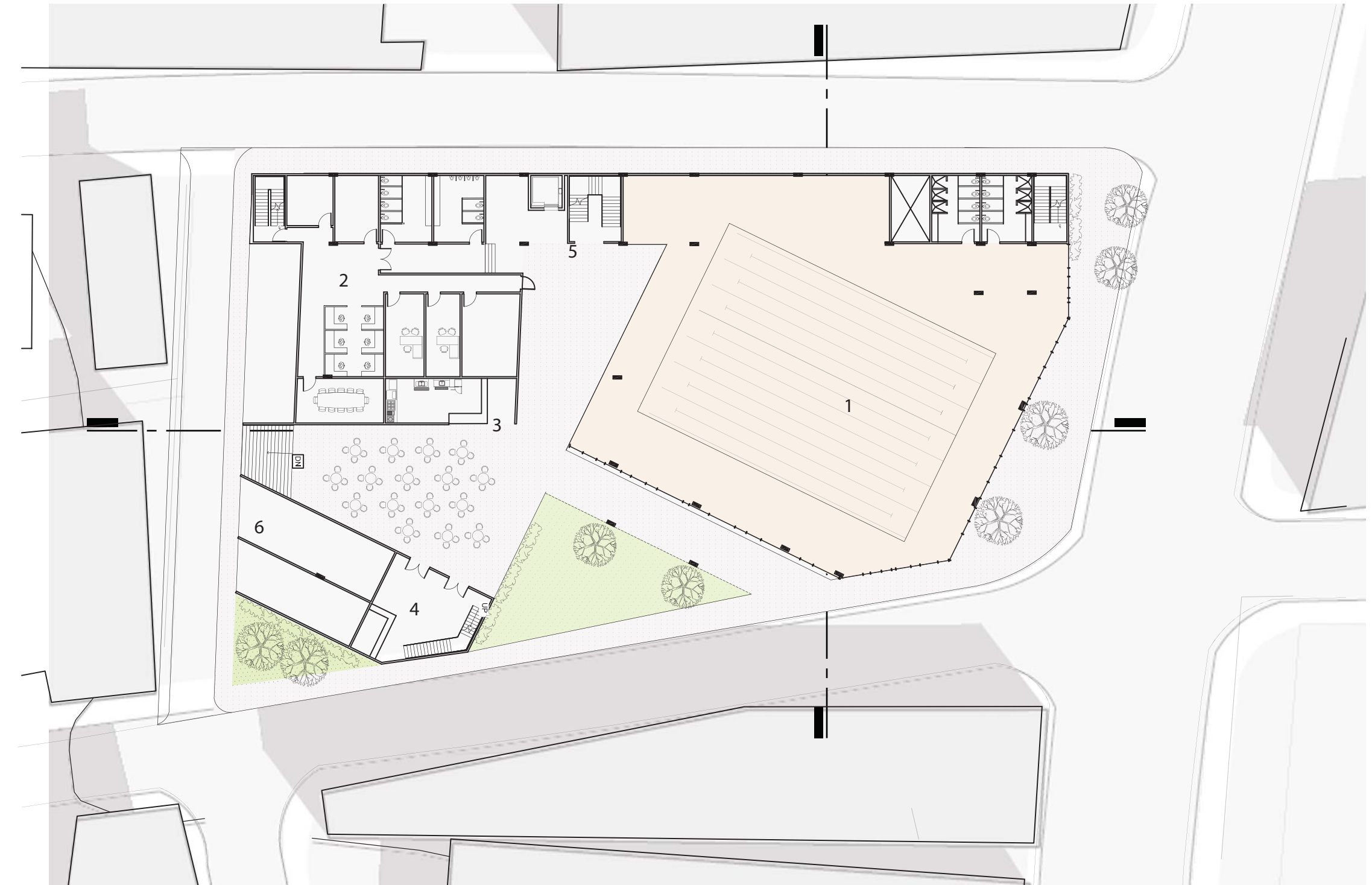
Planta Nivel 0 1/32"=1'-0" 1 Piscina 2 Oficinas 3 Cafetería 4 Tiendita 5 Acceso Principal 6 Acceso al Estacionamiento
